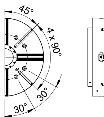
Fig. 7-1 : Série VT-S [Sous réserve de modifications techniques]
