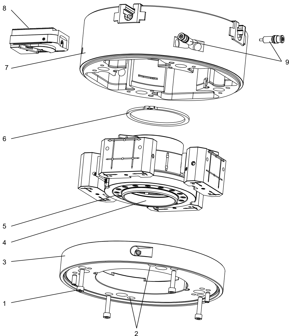
Fig. 5-2 : Démonter/monter le mandrin de serrage (VT-S 013 à VT-S 080)
