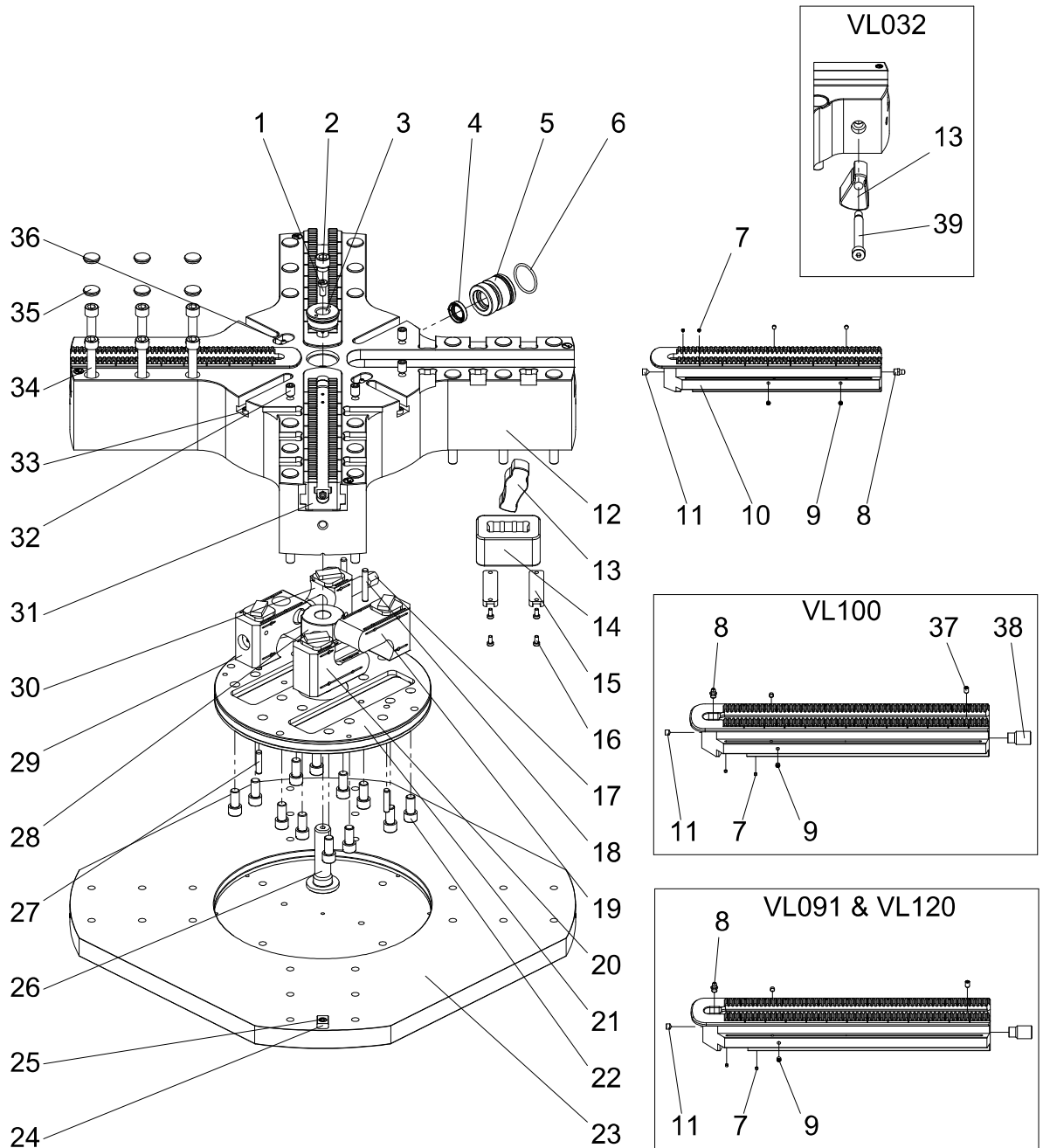
Fig. 8-1: Ricambi INOFlex® VL032 – VL120
