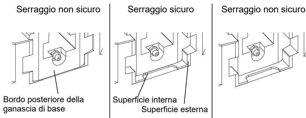
Fig. 4-2: Limitatore corsa
