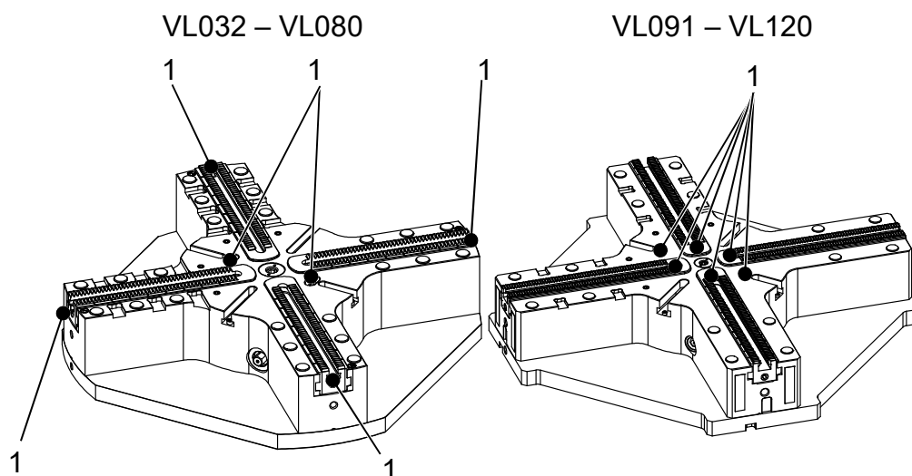
Fig. 5-1: Nippoli di lubrificazione
