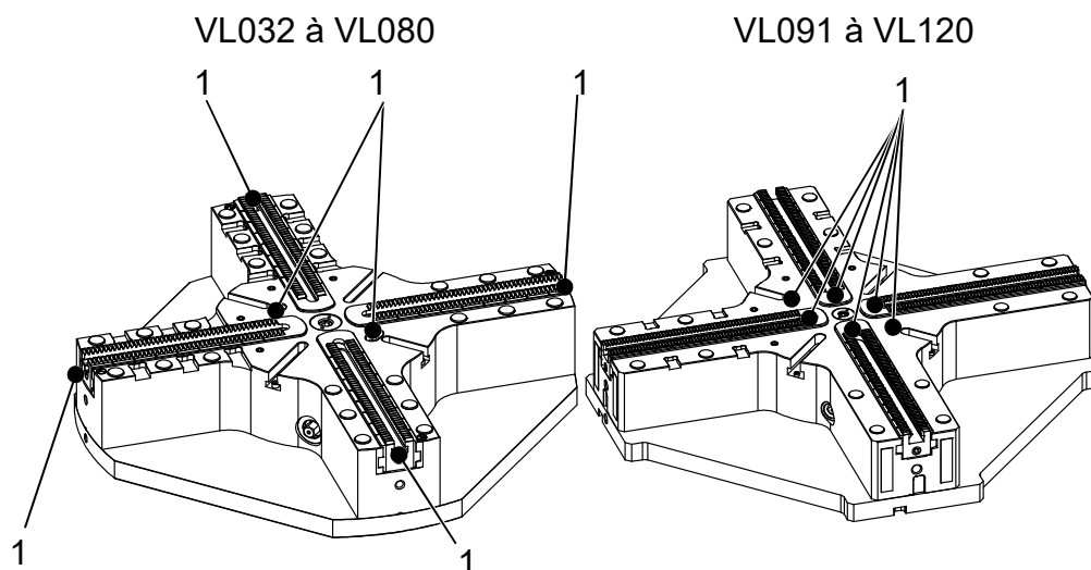
Fig. 5-1 : Graisseur
