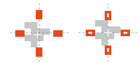
Zentrisch ausgleichende Spannung von geometrisch unregelmäßigen Teilen Concentric compensating clamping of geometrically irregular shaped parts
